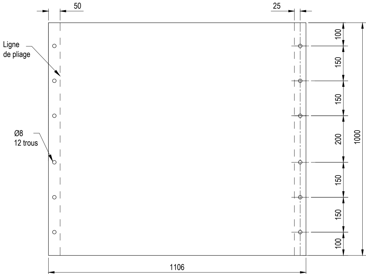
Vue déployée
