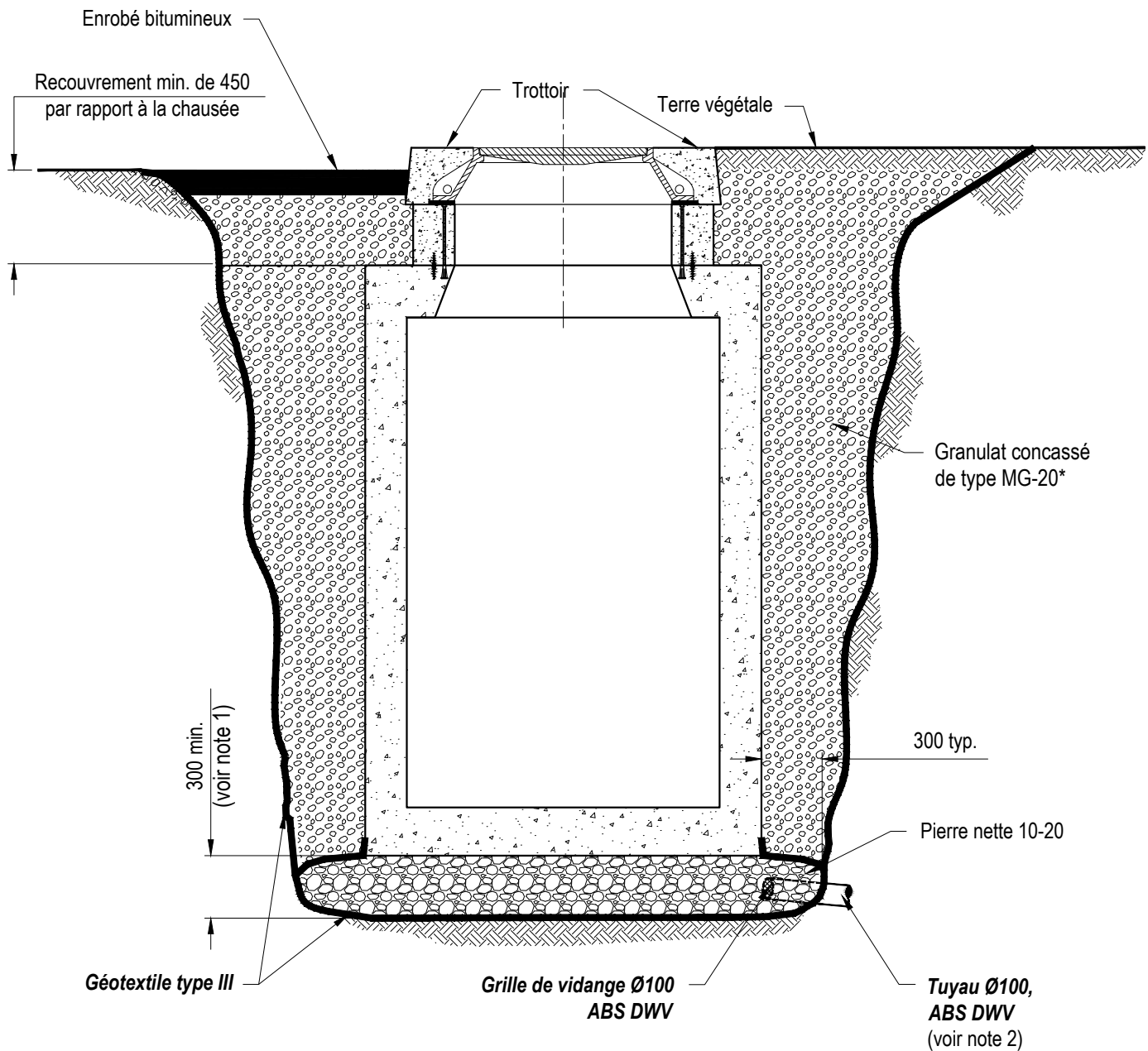
Vue en élévation
