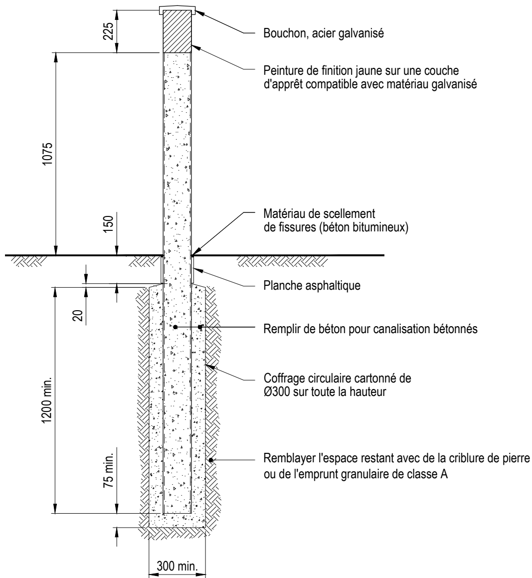
Vue en élévation
