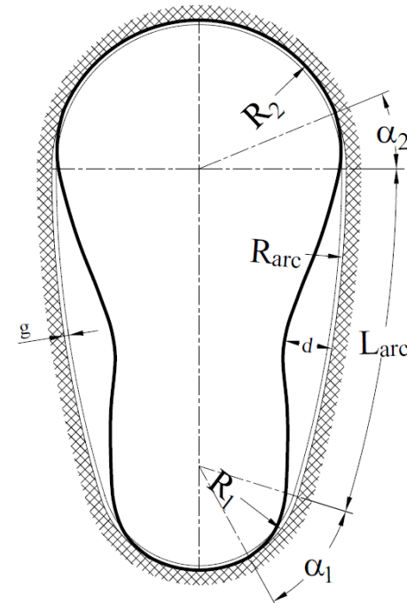
Profils à 3 rayons de courbure
